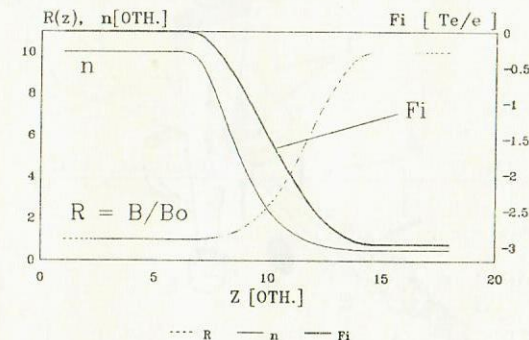
Рис. 2. Схема формирования потенциального барьера для электронов.
