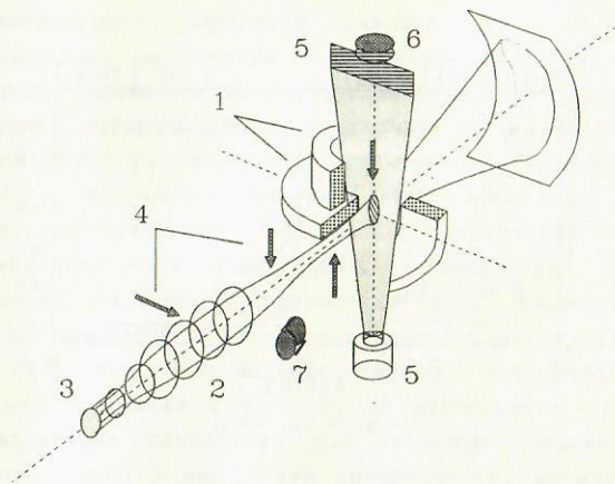
Рис.3. Схема установки «АМБАЛ - ЮМ»
