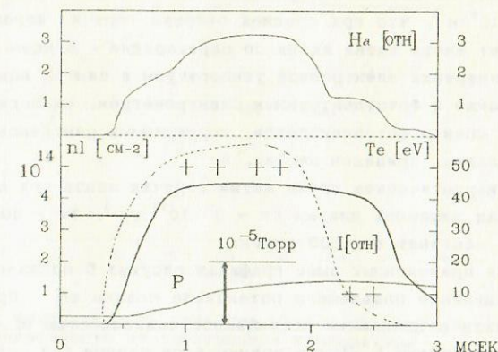
Рис. 6. Зависимости от времени в центре ловушки: давления газа, линейной плотности плазмы (жирная линия), температуры электронов (+) и интенсивности излучения на линии Na. Ток разряда источника - пунктирная линия.
