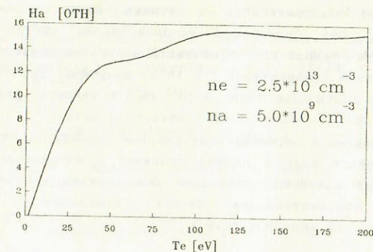
Рис. 7. Интенсивность свечения плазмы на линии \text{H}\alpha в зависимости от электронной температуры
