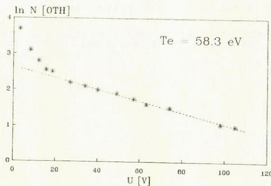
Рис. 8. Спектр рентгеновских фотоэлектронов.
