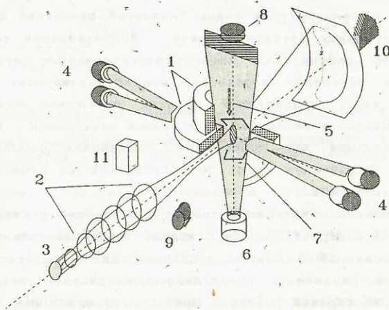
Рис.2. Схема установки «АМБАЛ - ЮМ»
