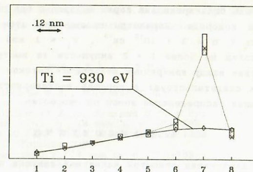
Рис. 11. Доплеровские измерения ионной температуры.
