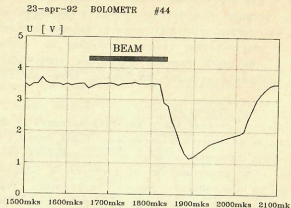
Рис. 7. Сигнал с болометра при работе пучков. ( отрицательная полярность )
