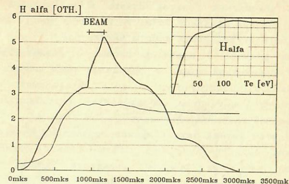
Рис. 8. Интенсивность свечения плазмы на линии H\alpha . Жирная линия - с атомарными пучками, пунктирная - без пучков, тонкая - давление вблизи плазмы. На вставке зависимость интенсивности свечения от электронной температуры.
