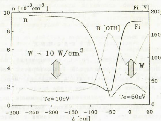
Рис. 1. Термобарьер, реализуемый на установке "Амбал-ЮМ"
