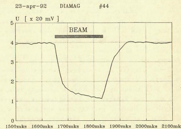
Рис.6. Диамагнитный сигнал при работе пучков.
