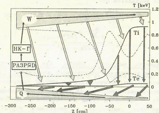
Рис.10. Диаграмма энергобаланса
