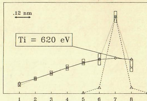
Рис.5. Доплеровские измерения ионной температуры.
