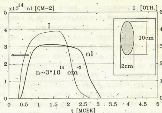
Рис. 3. Плотность плазмы в центре ловушки.
