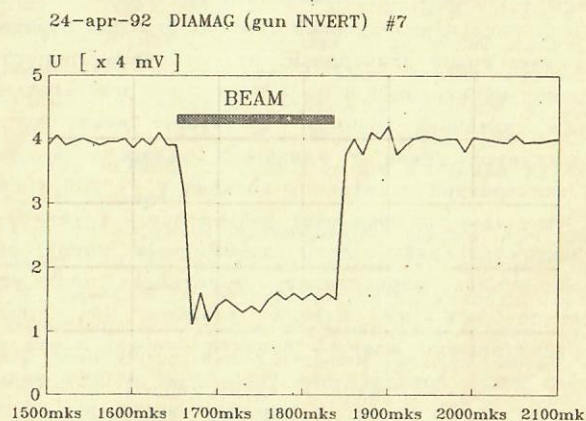
Рис.9. Диамагнитный сигнал при захвате пучков на плазменной струе с обращенным электрическим полем
